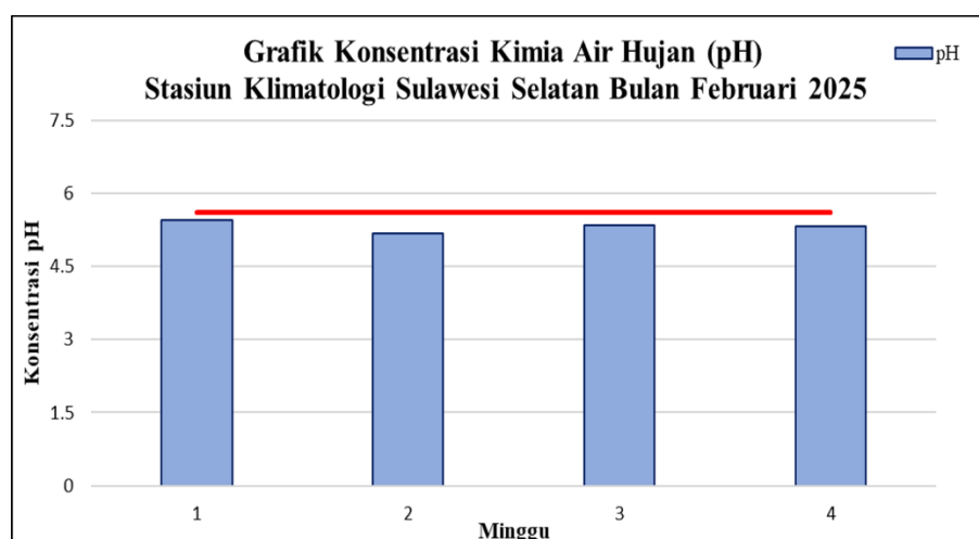
Gambar 25. Grafik Konsentrasi Kimia Air Hujan
